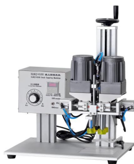
APM-XG-SC 半自动旋盖机 APM-XG-SC Semi auto screw capping machine
