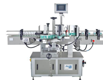
APM-LMR 全自动圆瓶贴标机 APM-LMR Automatic round bottle labeling machine
