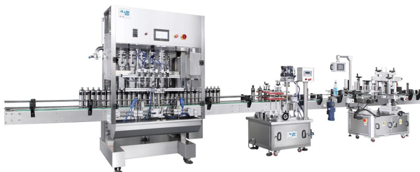
全自动液体灌装生产线 Automatic liquid filling production line
